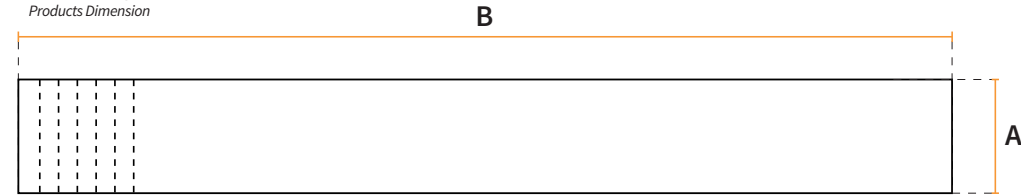
Khoanh cổ giấy (bề răng cưa - cắt vuông) Paper Collar Band (Square shape with dashed line)
