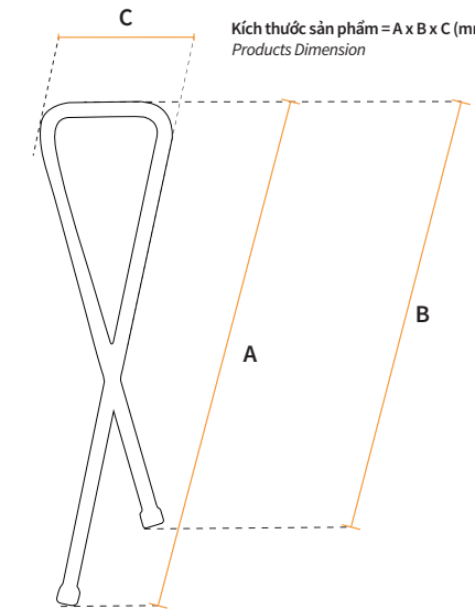
Model: Kẹp sắt tròn #02 Metal Shirt Clip #02
