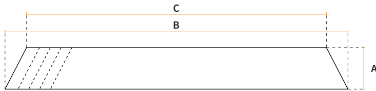
Khoanh cổ giấy (bề răng cưa - xéo góc) Paper Collar Band (Beveled edge with dashed line)
